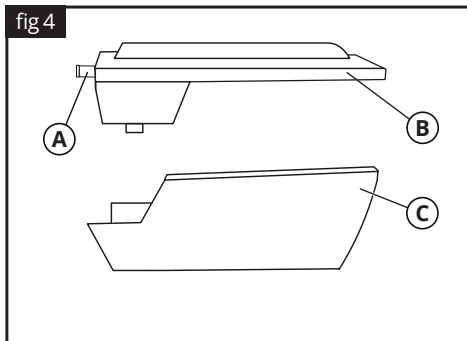
A. Locking tabs / Γλώσσες κλειδώματος B. Dust box (upper) / Δοχείο σκόνης (επάνω μέρος) C. Dust box (bottom) / Δοχείο σκόνης (κάτω μέρος)
